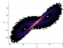
(d) Float16
